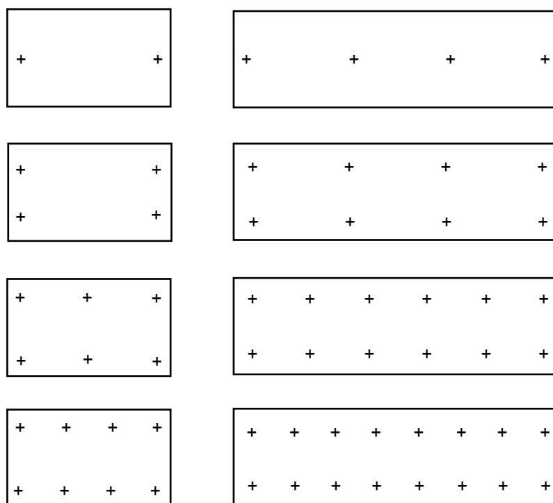
Fig. 1 : Plaatsingspatroon voor de mechanische bevestigingen (afstand : minimaal 100 mm van de rand in de lengterichting van de plaat en minimaal 150 mm van de rand in de breedterichting van de plaat)
